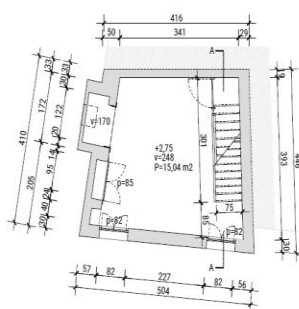
TLOCRT 1. KAT
