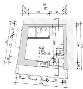
TLOCRT PRIZEMLJA
