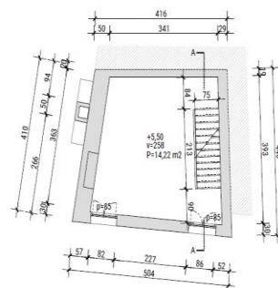
TLOCRT 2. KAT
